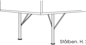
Stålbæn. H. 22
